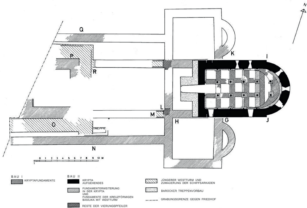
Abb. 11: Plan zur Ausgrabung im Bereich der Erasmuskapelle (nach Engemann 1972, 271).
