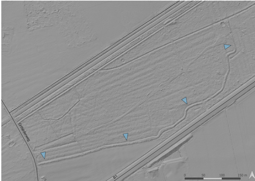
Abb. 7: Landwehr im Stadtbusch (Pfeile) im Digitalen Geländemodell (Quelle: GeoBasis NRW 2020; Bearb.: Altertumskommission für Westfalen/F. Jüngerich).
