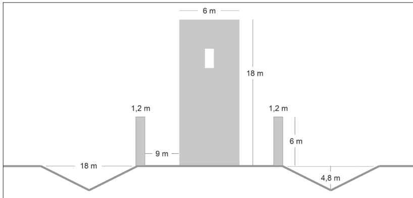
Abb. 14: Plan für den Bau von Warten aus dem Jahr 1429 (Grafik in Anlehnung an H. Rüthing 2002, 13).
